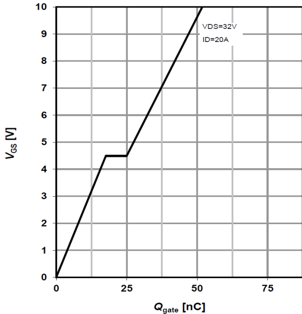
Typ.gate charge
