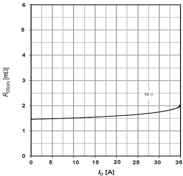
RDS(on) -- ID
